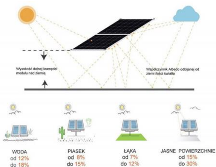
Rys. 1. Sposób działania modułu dwustronnego (bifacjalnego) - SolarInnova 5 .
